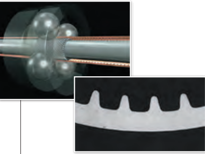
リップルフィンチューブ (R/F) 溝を持ったプラグを銅管に挿入し、外周のボールを高速回転させながら押し付け、銅管内面に溝を連続的に加工します。
