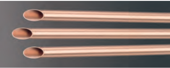
リップルフィンチューブ (R/F) 溝を持ったプラグを銅管に挿入し、外周のボールを高速回転させながら押し付け、銅管内面に溝を連続的に加工します。
