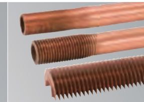
ローフィン、ミドルフィン、ハイフィン
