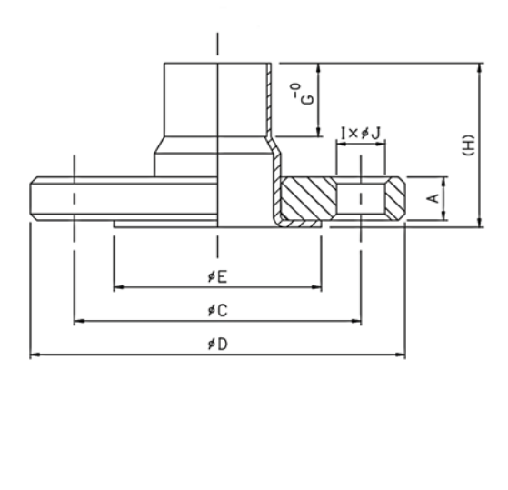
STC NC-F 10KG<セット> (単位mm)
