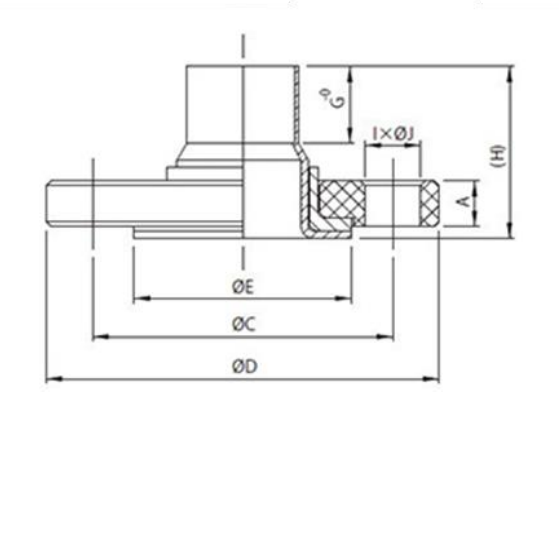
STC ZSF 10KG<セット> (単位mm)
