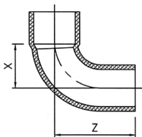
異径 90° エルボ
